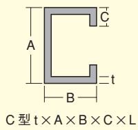
C型チャンネル
