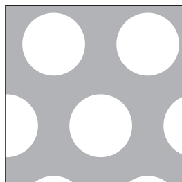
929338 生地 929738 シルバー AL 1×1 m×2 m 12φ×18P 929348 生地 929748 シルバー AL 1.5×1 m×2 m 12φ×18P 929362 生地 929762 シルバー AL 2×1 m×2 m 12φ×18P
