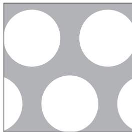
929363 生地 929763 シルバー AL 2×1 m×2 m 15φ×20P
