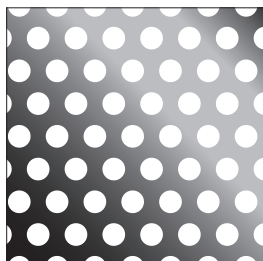
929480 SUS 2×1 m×2 m 3φ×5P BA 929490 SUS 3×1 m×2 m 3φ×5P 2B 929851 SUS 0.8×4'×8' 3φ×5P BA 929855 SUS 1×4'×8' 3φ×5P BA 929858 SUS 1.2×4'×8' 3φ×5P BA 929862 SUS 1.5×4'×8' 3φ×5P BA
