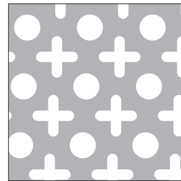
929324 生地 AL 0.5×1 m×2 m ○×+ 929328 生地 929728 シルバー AL 0.8×1 m×2 m ○×+ 929339 生地 929739 シルバー AL 1×1 m×2 m ○×+ 929350 生地 929750 シルバー AL 1.5×1 m×2 m ○×+
