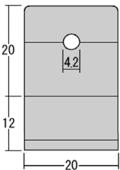
TB壁面固定金具シルバー
