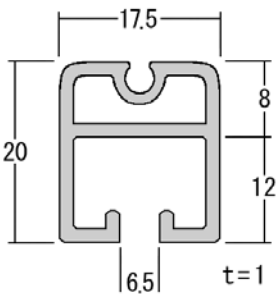
TB-MフレームX4mシルバー
