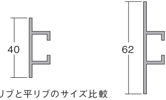
小リブと平リブのサイズ比較
