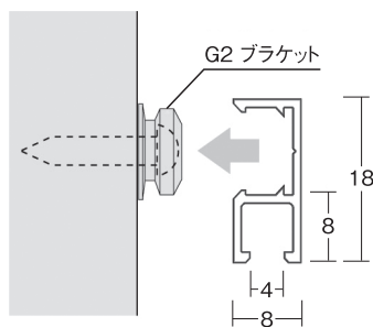
G-2 部品セット
