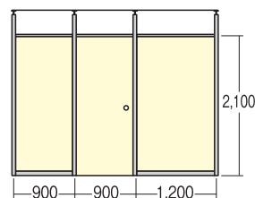
NF-1 型 密閉タイプ
