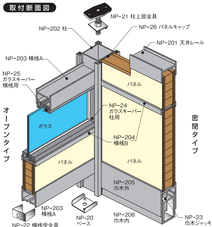
NS-101 型 オープンタイプ
