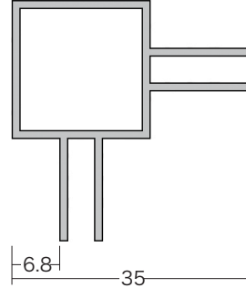
1000131 シルバー アルミコネクター FJ - 3
