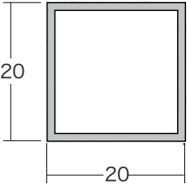
12019 シルバー □ 1.5 × 20 × 20 × 4 m
