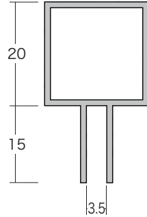
1000121 シルバー アルミコネクター FJ - 2
