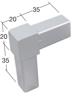
1000111 シルバー アルミコネクター FJ - 1
