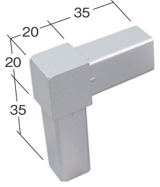
1000111 シルバー アルミコネクター FJ - 1
