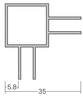
1000131 シルバー アルミコネクター FJ - 3
