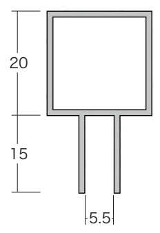
1000121 シルバー アルミコネクター FJ - 2
