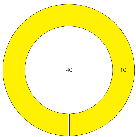
951161 発泡カバー 丸 40 φ 用 × 0.9 m イエロー
