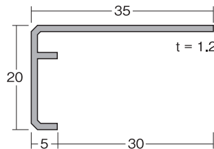
220501 看板枠 39609 × 3.64 m シルバー
