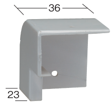
908152 プラコーナー グレー 看板枠 39609 用
