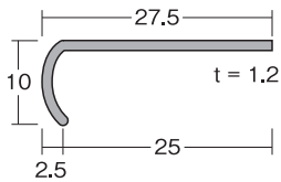
220500 看板枠 35463 × 3.64 m シルバー
