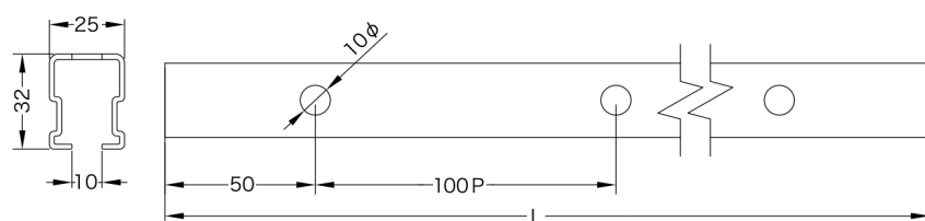
912403 シーリングバー 1,800L
