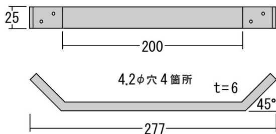
1000207 シルバー FB6X25 トラスブラケット
